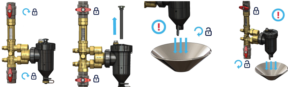
Рис. 16. Схема технического обслуживания AHS 560
