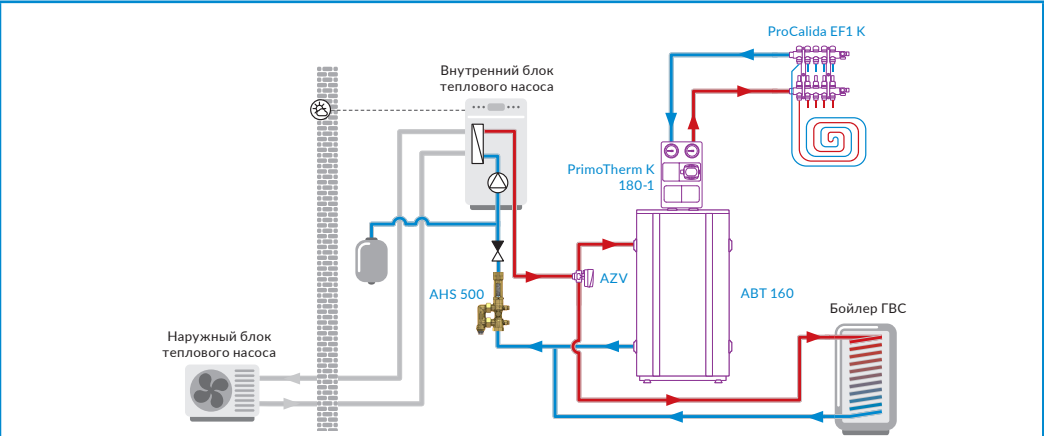
Рис. 12. Пример схемы монтажа с комплектом сервисной арматуры для тепловых насосов AHS 500
