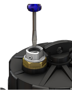
Рис. 11. Открытие ручного воздухоотводчика
