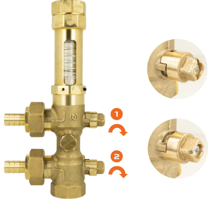
Рис. 4. Запорные клапаны в корпусе AHS
