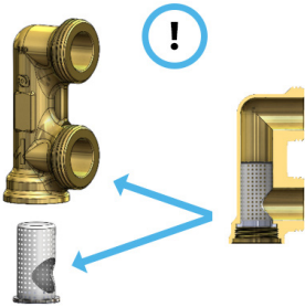
Рис. 15. Правильное расположение сетчатого фильтра
