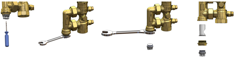
Рис. 14. Схема технического обслуживания AHS 500
